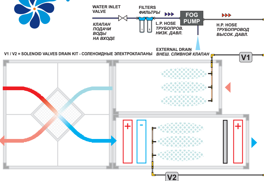
Типичная схема монтажа АКВ: Увлажнение и предварительное охлаждение AHU Mounting layout example: Humidification and Pre-cooling
