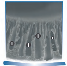
Фрагмент волокна Hollow fiber section
