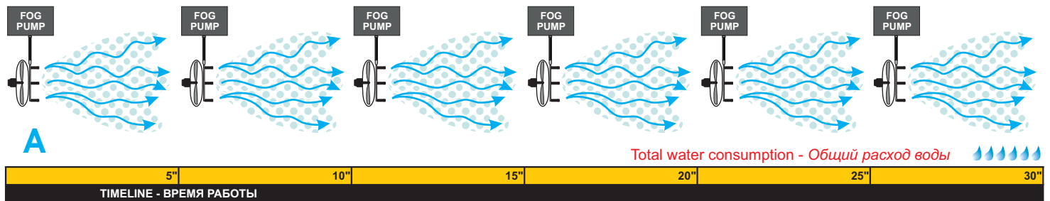
B) "TIME" version pump with 5" ON / 5" OFF mode setting - Насос с системой "TIME" в режиме 5 с работа / 5 с пауза
