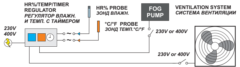
Панель управления насосом и вентиляторами - 230V / 400V
